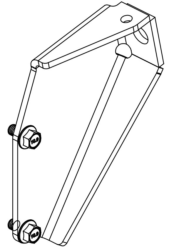
ISO VIEW ASSEMBLED SCALE: 2:3
